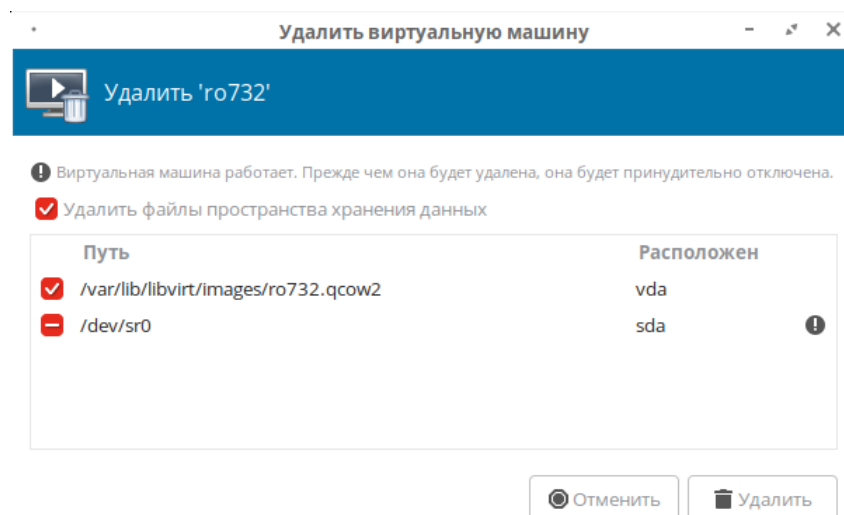
Рисунок 13.39 – Удаление ВМ
