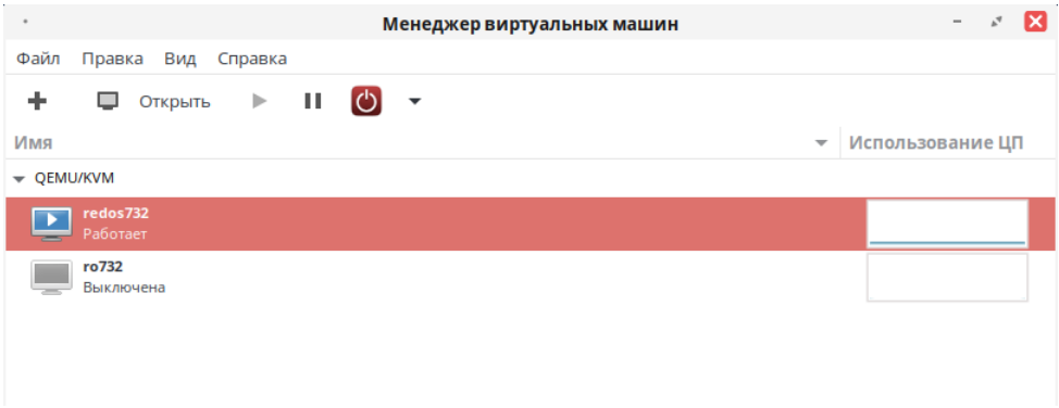
Рисунок 13.18 – Выбор ВМ
