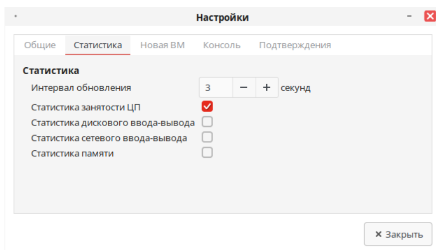
Рисунок 13.24 – Вкладка Статистика
